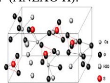
FIGURA 1 – Célula cristalina Fonte: CANUT, 2006, p. 30
